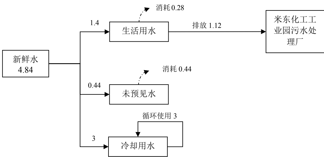
图 1 本项目给、排水平衡图（单位 t/d）
