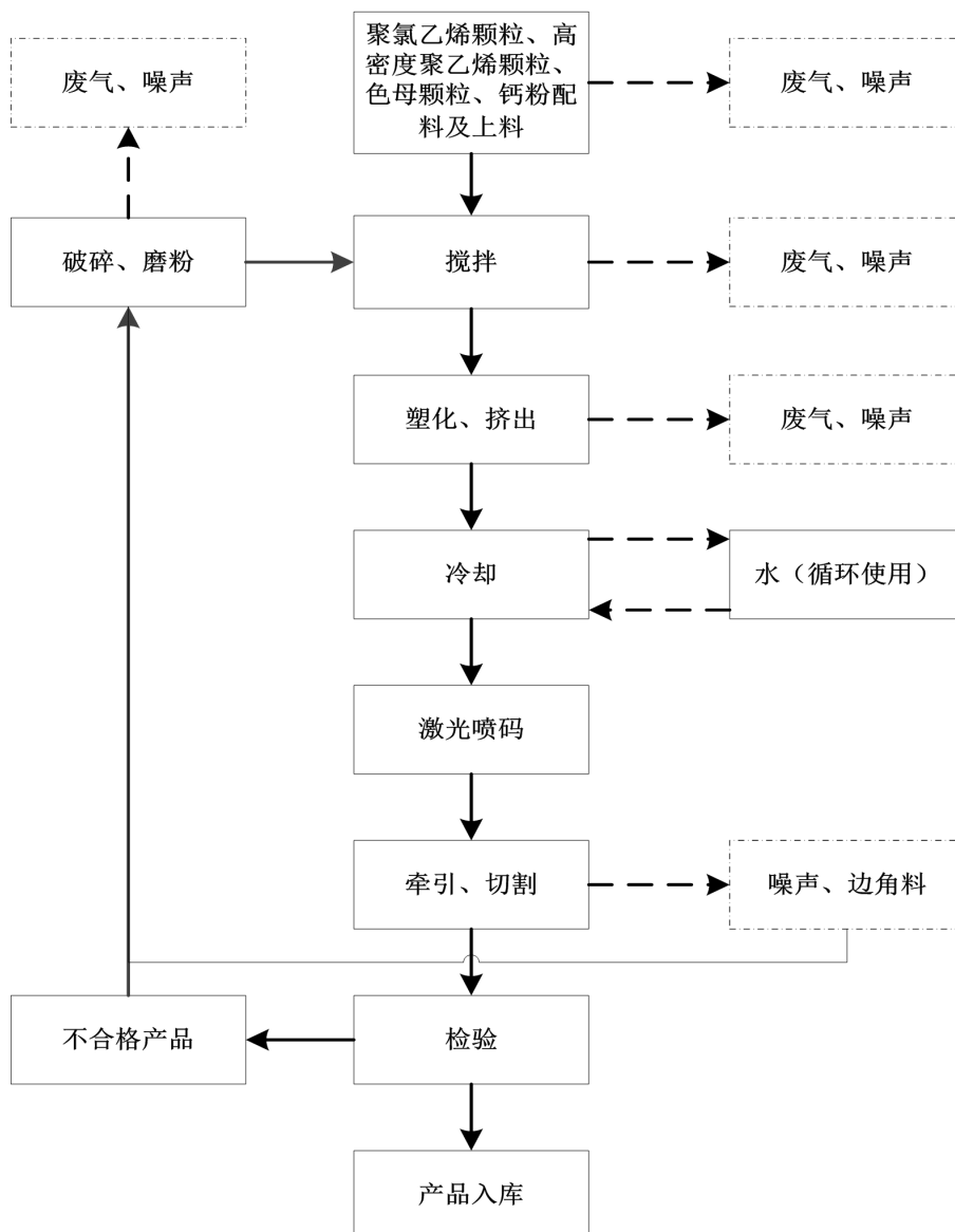
图3 运营期生产工艺流程及产污环节图
